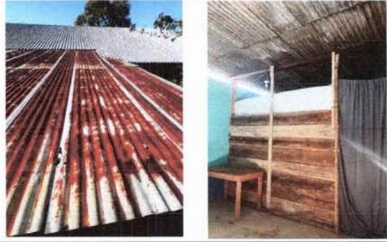
FOTO 2: Se observa el constante deterioro de lámina y la mala infraestructura del techo, lo que representa un constante riesgo
